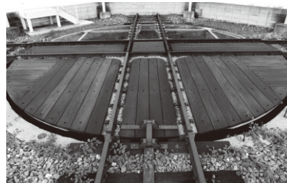
武豊停車場跡に残る転車台
